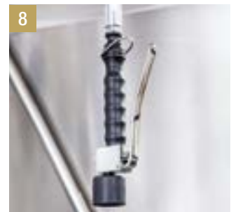
8 LOW-FLOW Brausekopf: Interne Komponenten und Wasserdurchgänge aus Edelstahl, Feststellring für Dauerbetrieb, Anti-Drop- und Anti-Leckvorrichtung.
